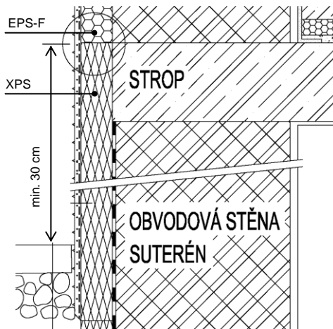
Obrázek 7: Sokl zateplený neuskočený
