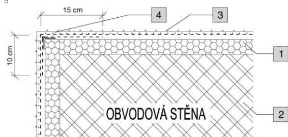
Obrázek 10: Varianta s rohovým profilem s integr. síťovinou
