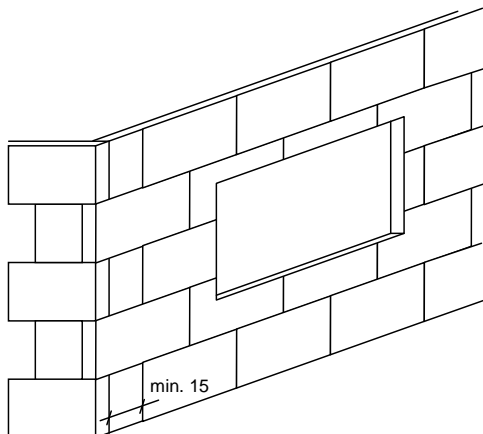
Obrázek 1: Kladení polystyrenových fasádních desek EPS-F
