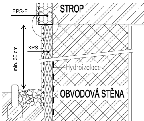
Obrázek 6: Sokl zateplený uskočený
