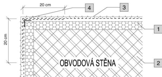
Obrázek 9: Varianta s rohovou lištou 9079
