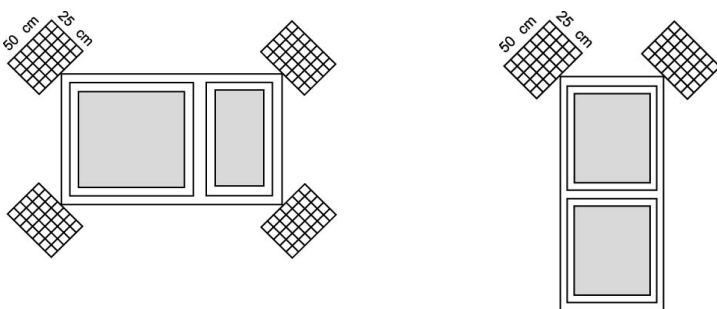
Obrázek 2 : Dodatečné vyztužení rohů oken a dveří
