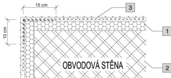
Obrázek 8: Varianta bez rohové lišty
